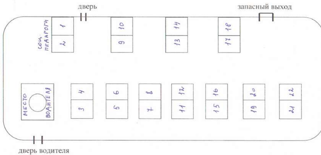
Схема посадочных мест в школьном автобусе
